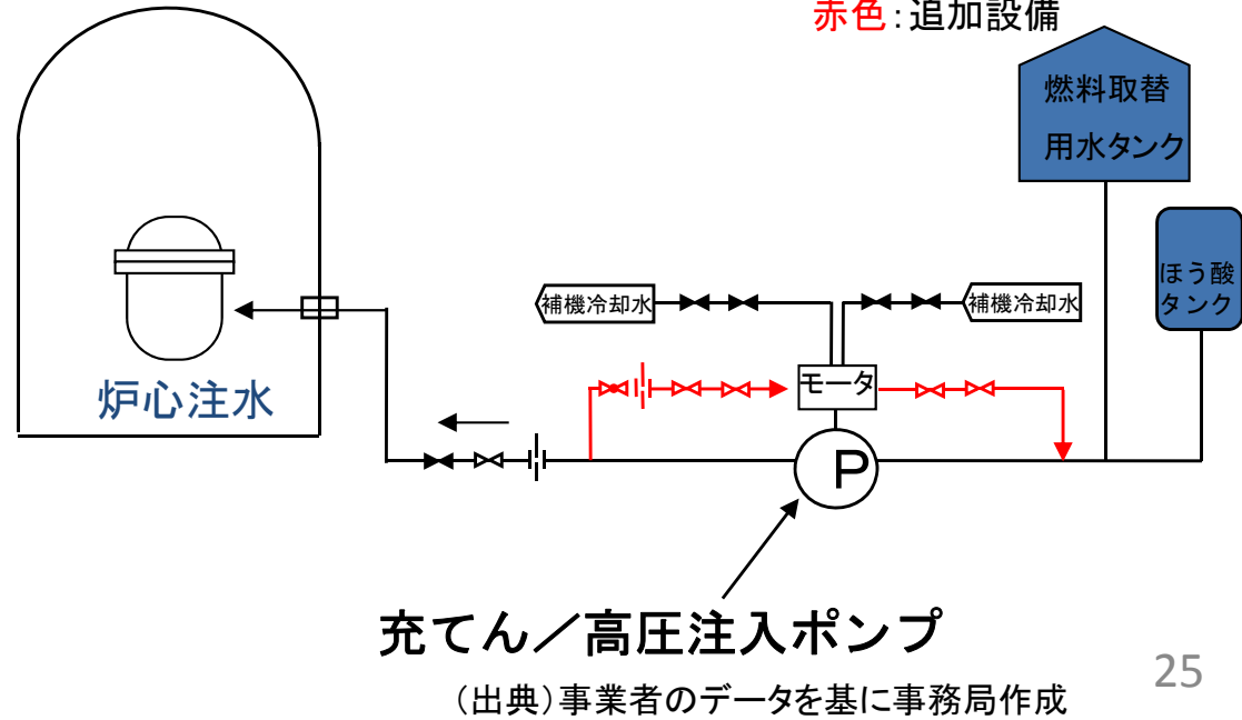
④-10 充てん高圧注入ポンプ自己冷却設備設置
