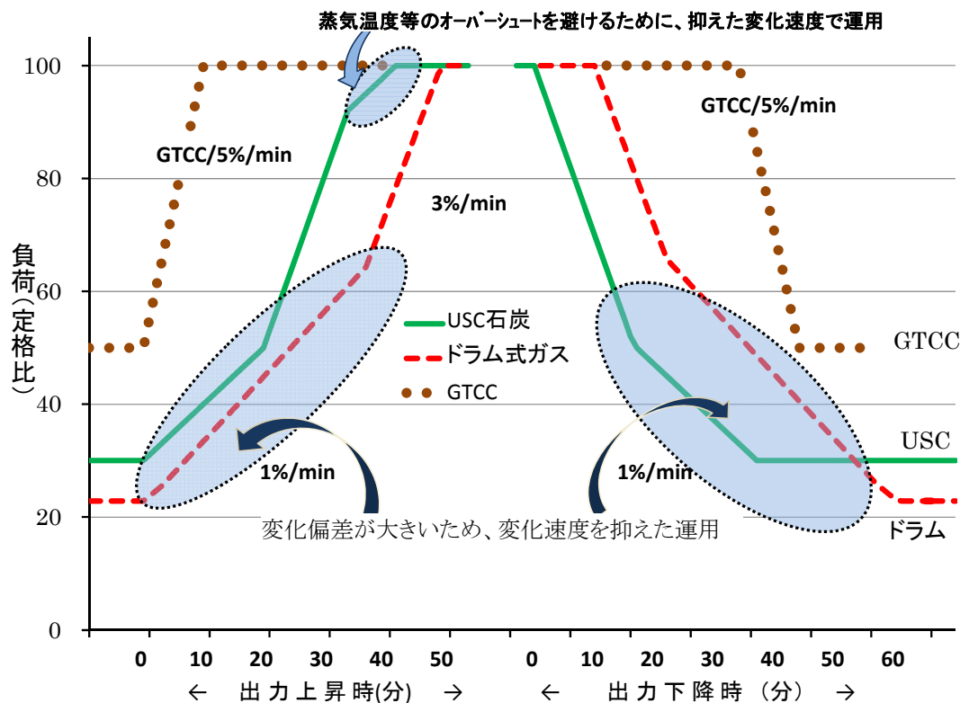
【火力プラントの出力変化の一例】
