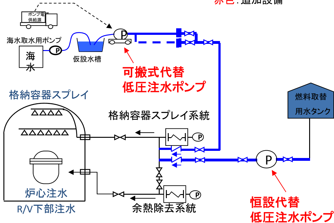
④-8 低圧注入用配管装置
