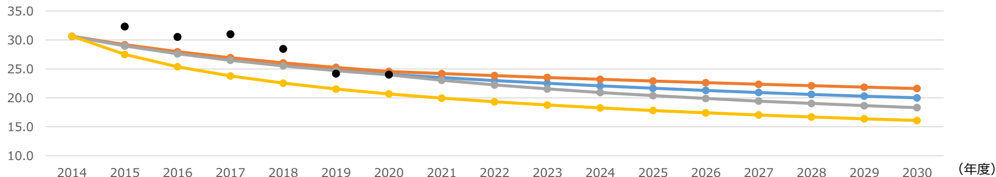
＜15年コスト検証委における設備費コスト予測と実績の比較【事業用】＞
