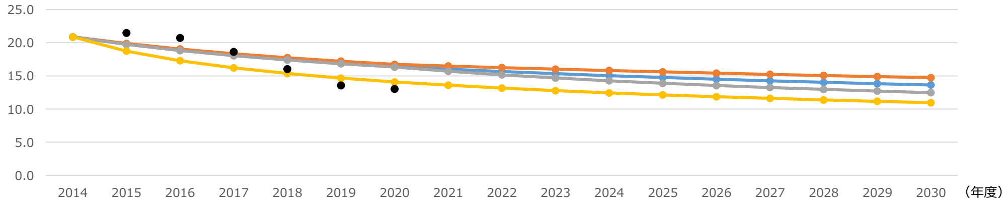
＜15年コスト検証委における設備費コスト予測と実績の比較【事業用】＞
