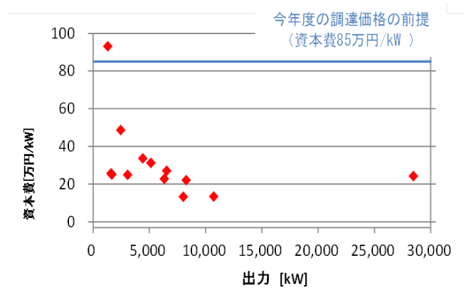
【参考 19】 中小水力発電 (1,000kW 以上) の出力と資本費の関係
