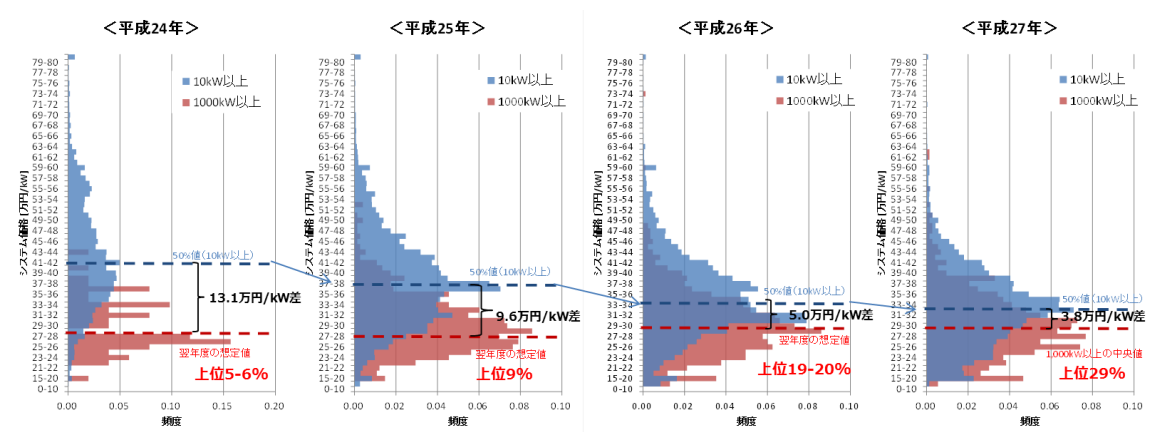
【参考 4】 10kW 以上全体・1,000kW 以上の太陽光発電のシステム費用分布（設置年別）
