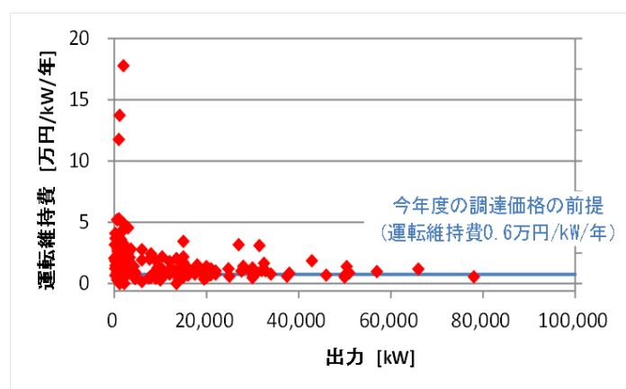
【参考 13】 陸上風力発電（20kW 以上） の出力と運転維持費の関係
