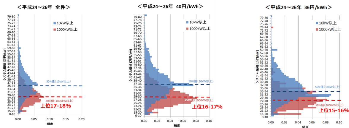
【参考 5】 10kW 以上全体・1,000kW 以上の太陽光発電のシステム費用分布（適用された価格別）
