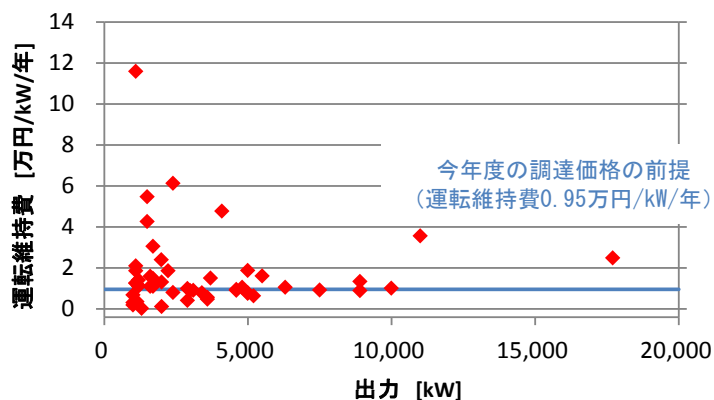
【参考 20】 中小水力発電 (1,000kW 以上) の出力と運転維持費の関係
