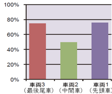
空気抵抗低減値(車間距離4m時)
