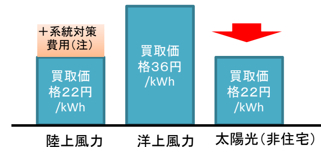
【風力発電及び太陽光発電導入に係る追加的費用(2030年度)】
