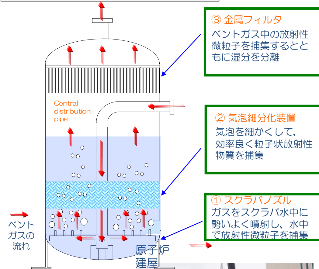
フィルタベント装置の概要
