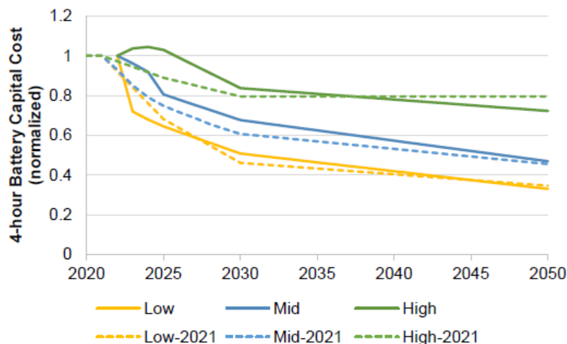
米国エネルギー省による4時間率の蓄電池コストの予測
