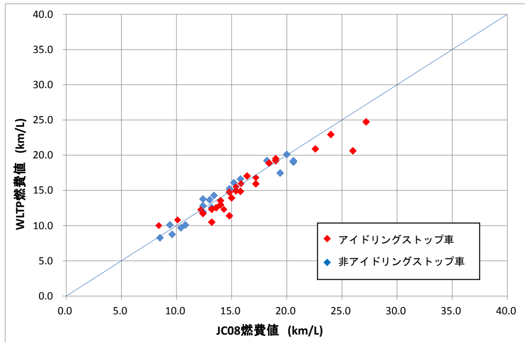
図3 軽乗用自動車やハイブリッド乗用自動車を除く乗用自動車における WLTP 燃費値と JC08 燃費値
