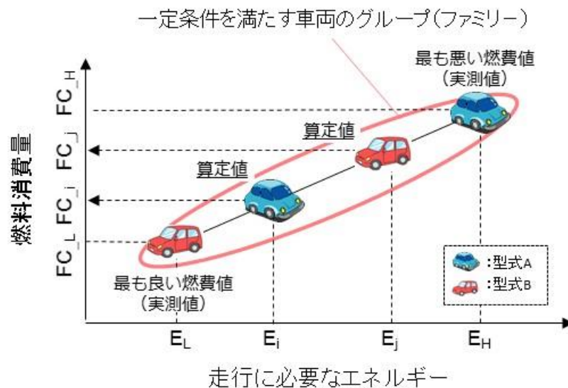
図 2 コンバインドアプローチ概念図
