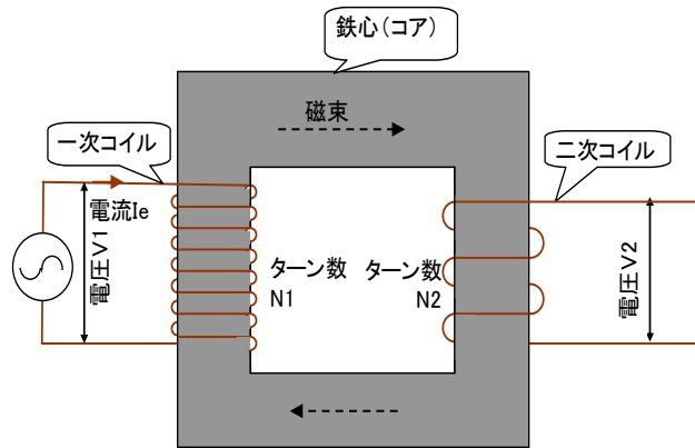
図 I. 5 変圧器の原理（無負荷時）
