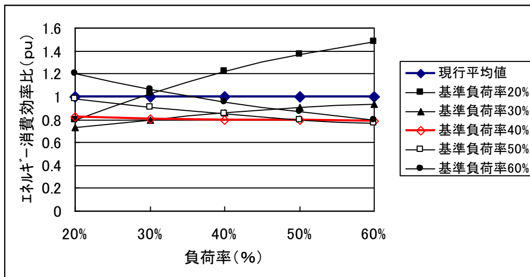
図2 最適負荷率別 負荷率－全損失特性
