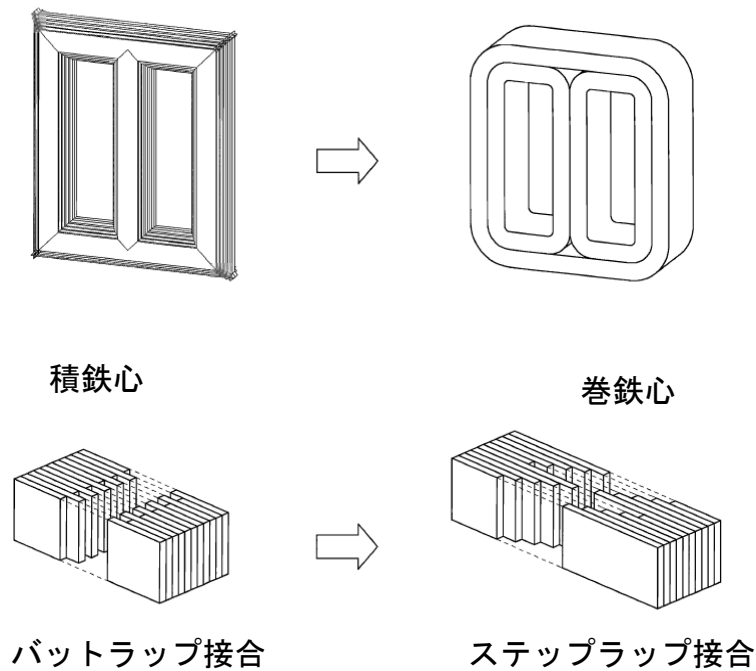
図 I. 8 鉄心構造の改良
