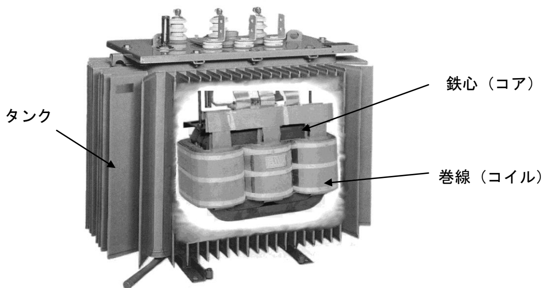
図 I . 3 油入変圧器の構造
