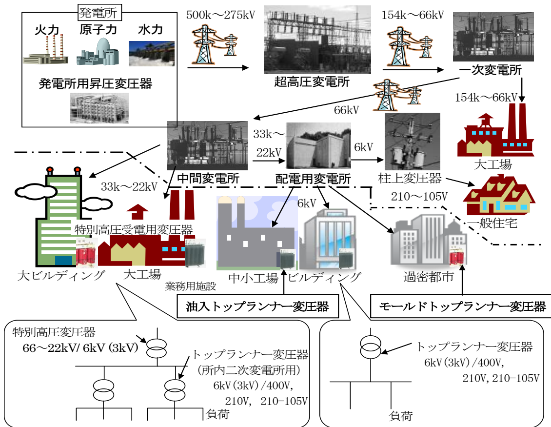
図 I.1 送配電系統概略図
