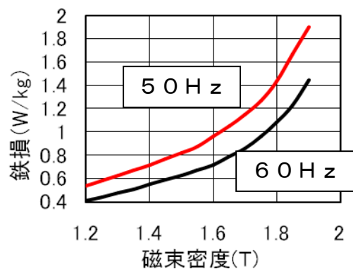
図 I. 9 電磁鋼板の鉄損特性例
