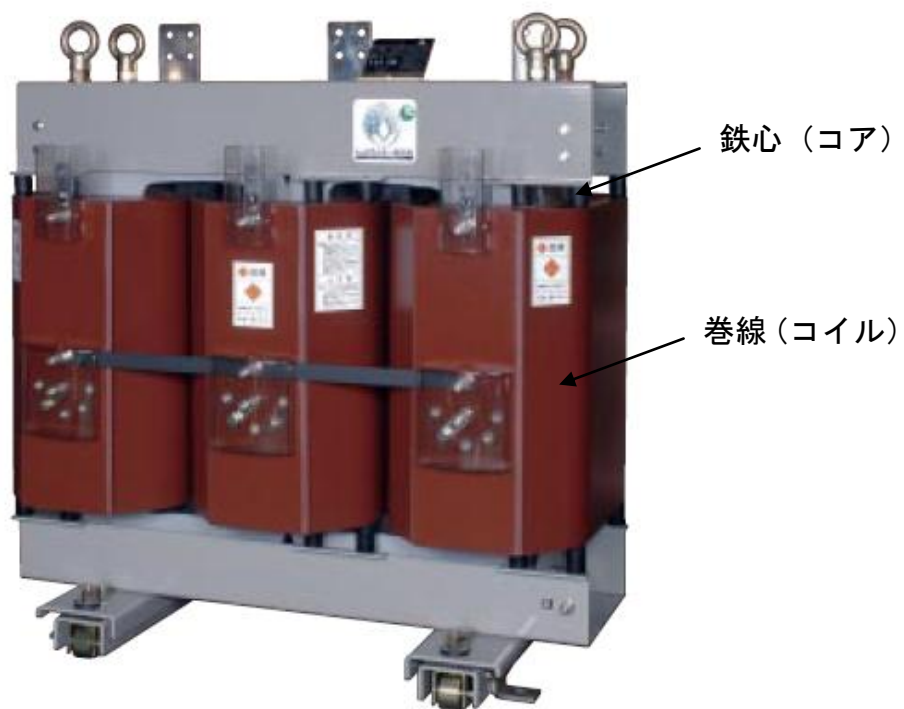
図 I . 4 モールド変圧器の構造
