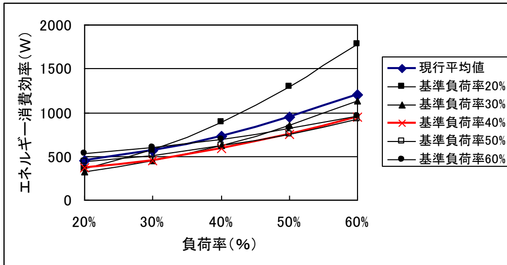
図1 最適負荷率別 負荷率－全損失特性
