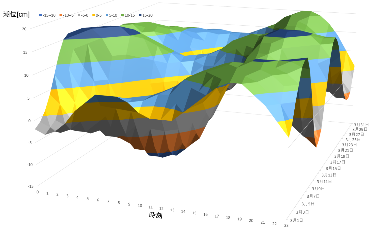
秋田港の潮位変化(2020/3/1～3/31)
