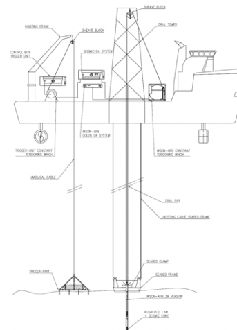
作業船
