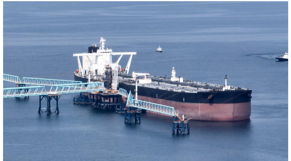
白島国家石油備蓄基地タンカー着岸作業の様子
