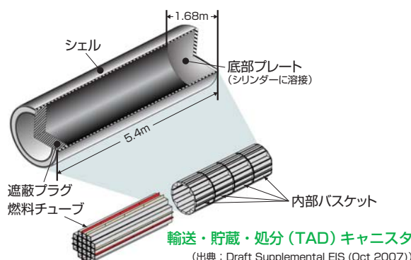
廃棄物パッケージの種類
