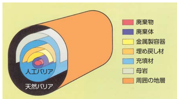
多重バリアシステムの考え方
