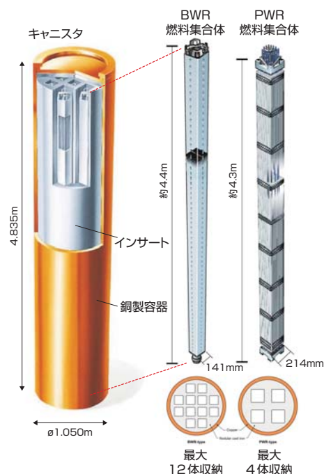
キャニスタへの使用済燃料の封入
