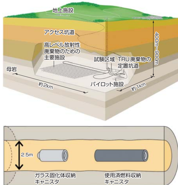
オパリナス粘土層内での高レベル放射性廃棄物の処分場とキャニスタの定置イメージ
