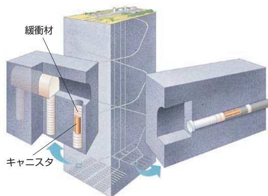
KBS-3 処分概念
