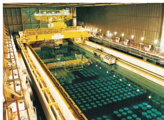
酸化燃料再処理プラント（THORP）内の 使用済燃料貯蔵プール (セラフィールド社ウェブサイトより引用)
