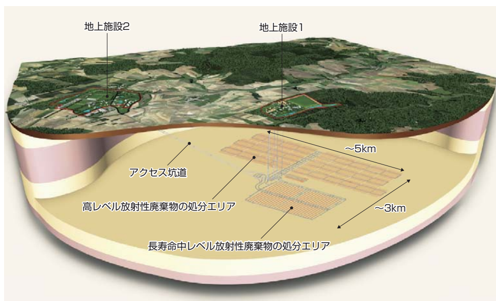
フランスにおける処分場の概念図
