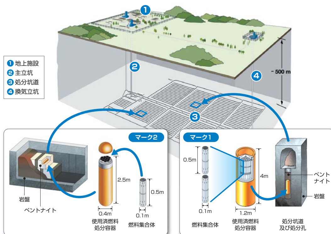
地層処分場の概念図
