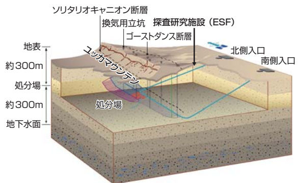
ユッカマウンテン処分場の全体レイアウト
