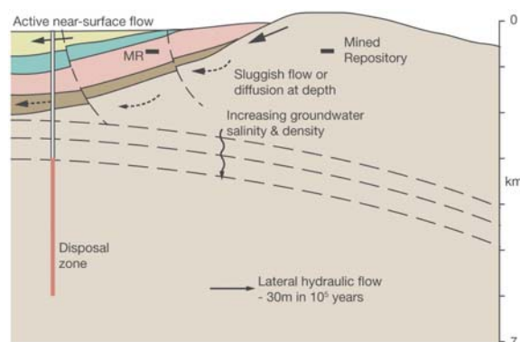
超深孔処分概念
