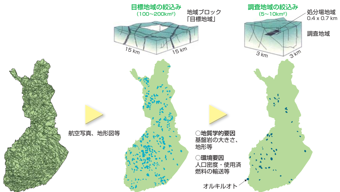
サイト確定調査（1983～1985年）における調査地域の選定・絞り込み
