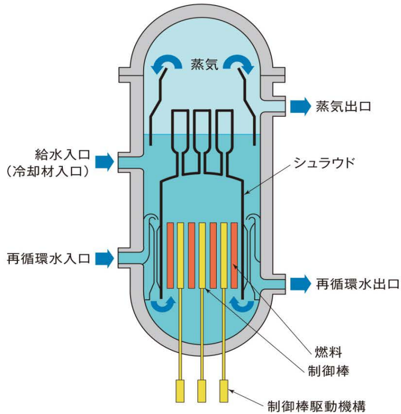
沸騰水型原子炉 (BWR)
