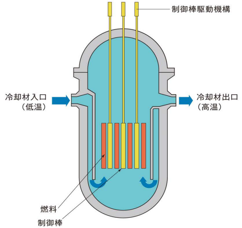
加圧水型原子炉 (PWR)
