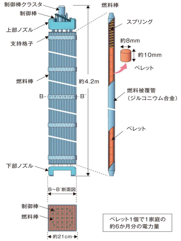
加圧水型炉 (PWR) の燃料集合体
