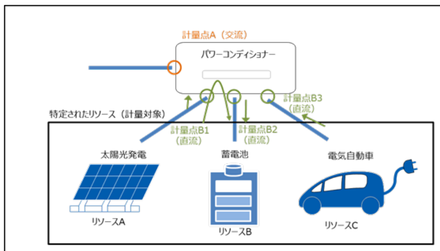
図 12：マルチ入力 PCS の潮流例
