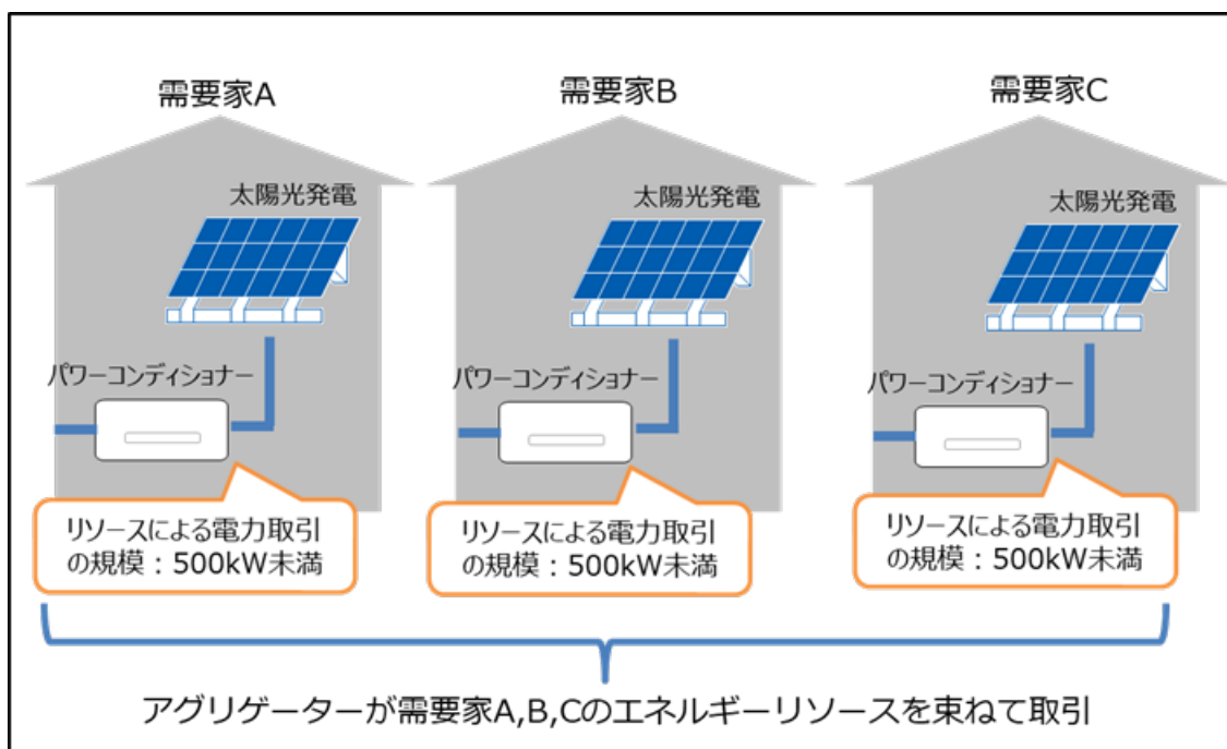
図 17：アグリゲーター等が特定計量をする場合の電力の規模 500kW の考え方
