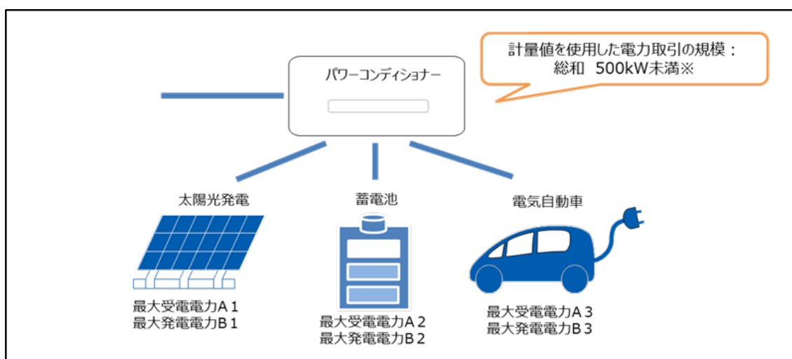
図 15：複数のリソース等を 1 つの電気計器（マルチ入力 PCS）で束ねて計量する場合の電力の規模 500kW の考え方
