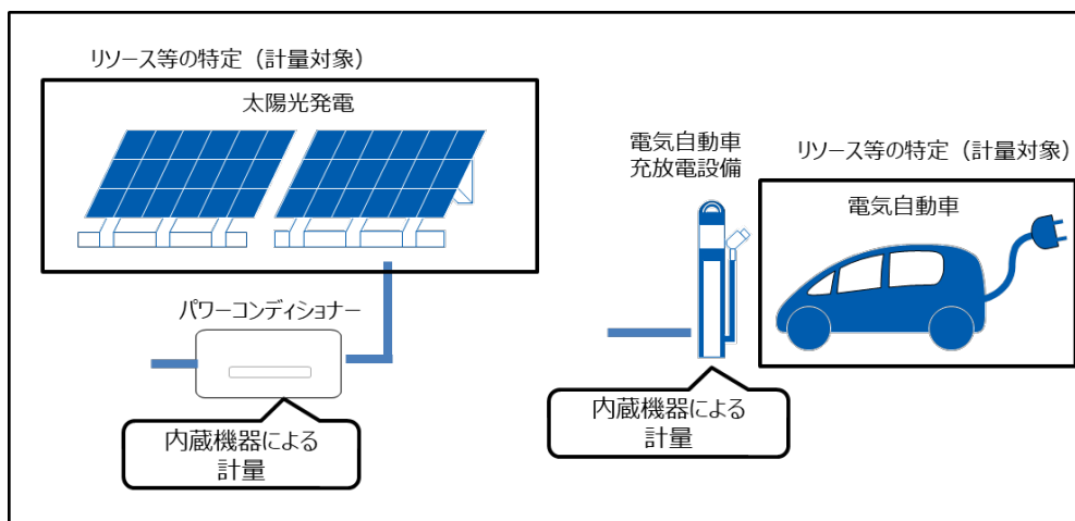
図1: リソース単位で計量する電力量を特定するイメージ
