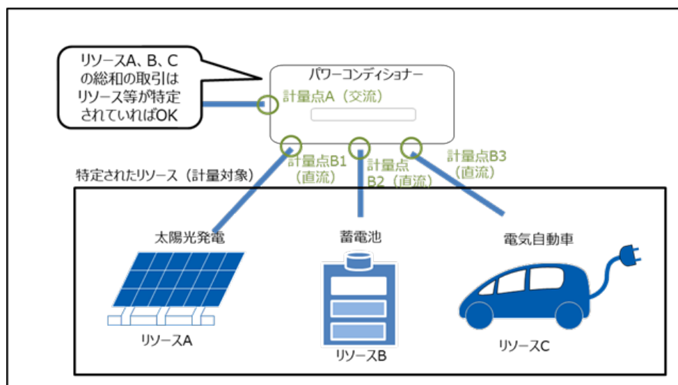
図4：マルチ入力 PCS を使用した取引等について
