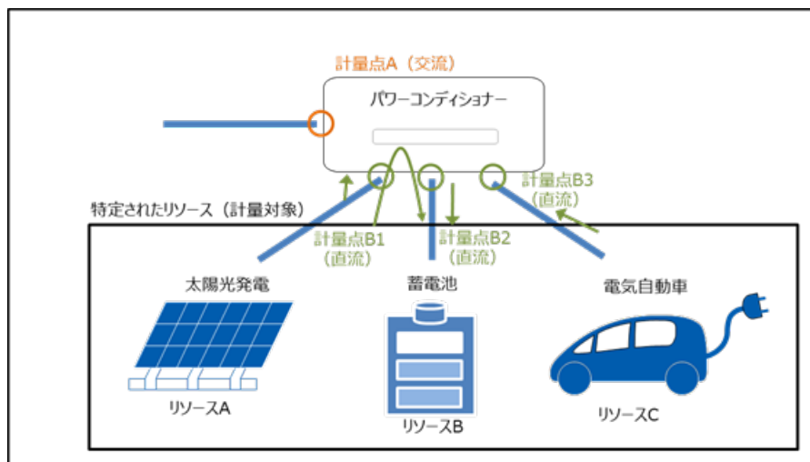
図 13：マルチ入力 PCS の潮流例（再掲）
