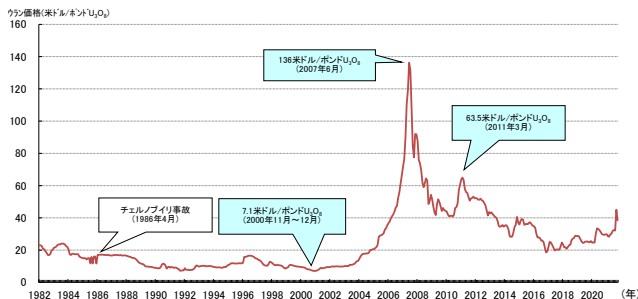
【第222-2-7】ウラン価格(U 3 O 8 ) 11 の推移
