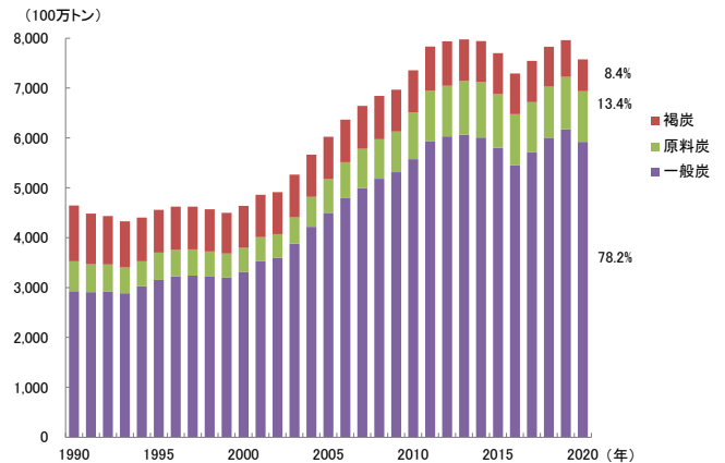
【第222-1-33】世界の石炭生産量の推移(炭種別)
