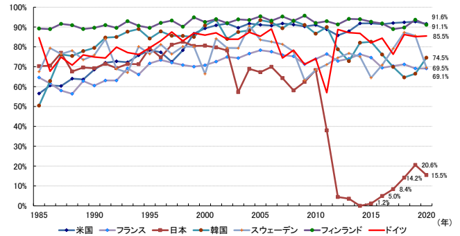
【第222-2-3】主要原子力発電国における設備利用率の推移
