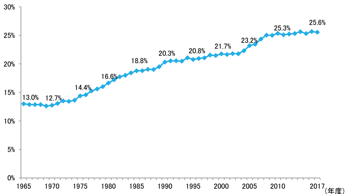
【第211-3-3】電力化率の推移
