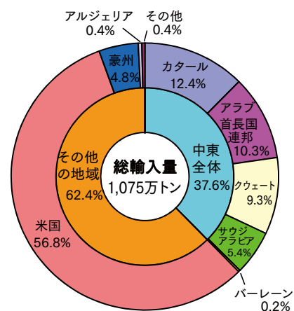
【第213-1-16】LPガスの輸入先(2017年度)
