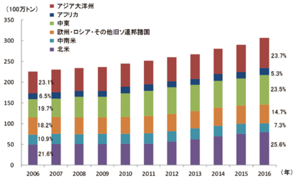
【第222-1-26】世界のLPガス地域別生産量
