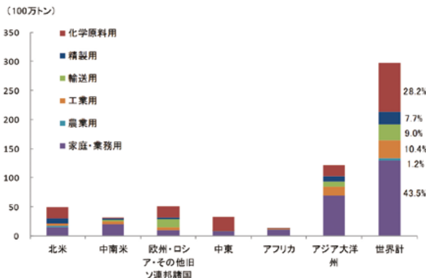
【第222-1-28】世界のLPガス用途別消費量(2016年)
