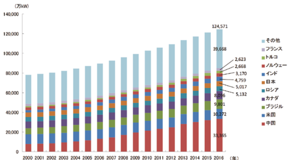
【第222-2-14】世界の水力発電の導入状況
