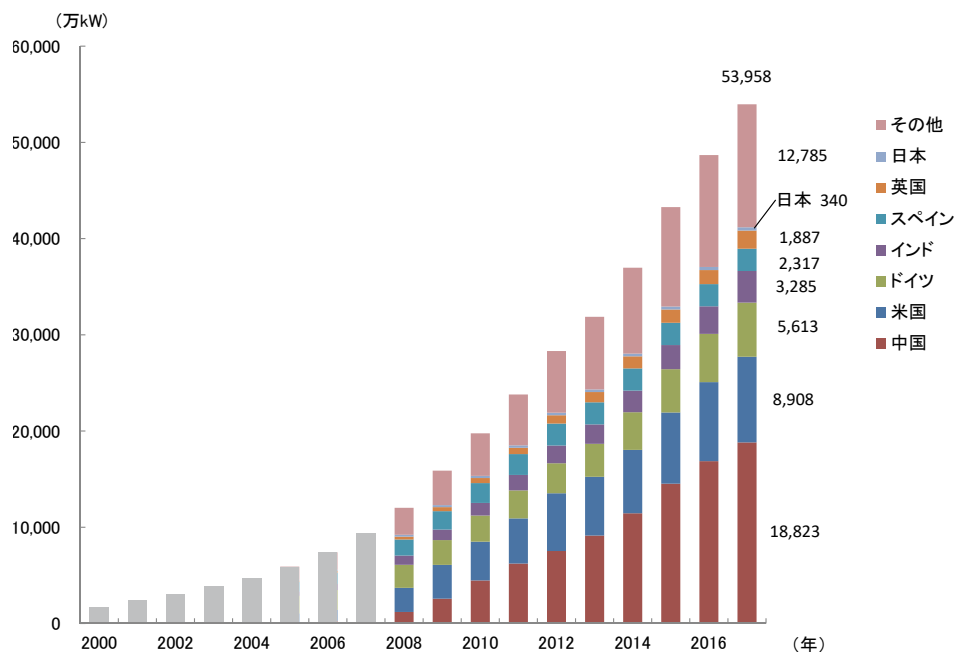
【第222-2-12】世界の風力発電の導入状況
