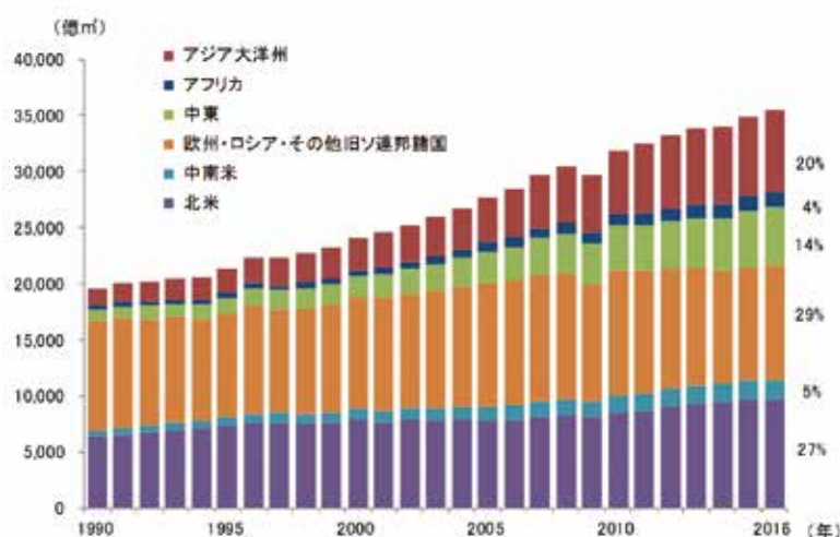
【第222-1-17】天然ガスの消費量の推移(地域別)
