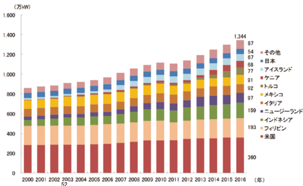
【第222-2-15】世界の地熱発電設備
