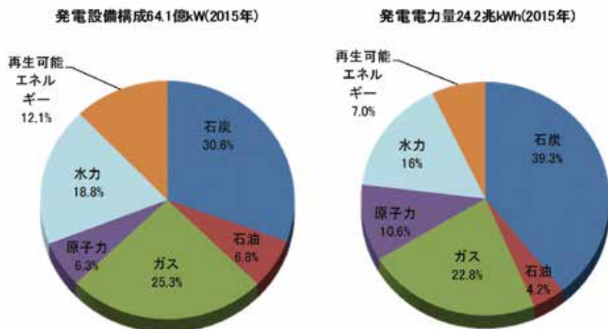
【第223-1-5】世界の電源設備構成と発電電力量
