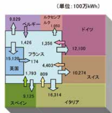
【第223-1-7】欧州の電力輸出入の状況(フランスの例、2015年)
