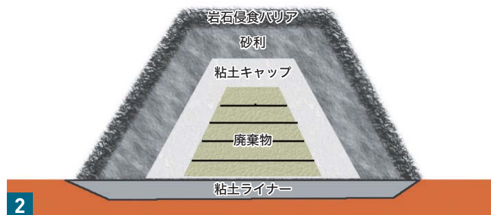
1 クライブ処分場の敷地レイアウト 2 処分セルの断面イメージ図
