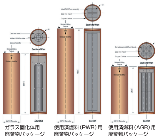
ガラス固化体と使用済燃料の処分パッケージ案 （出典：NDA/RWMD/054）
