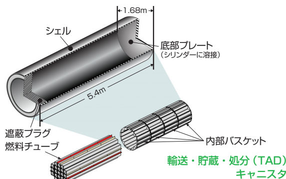
輸送・貯蔵・処分 (TAD) キャニスタ
