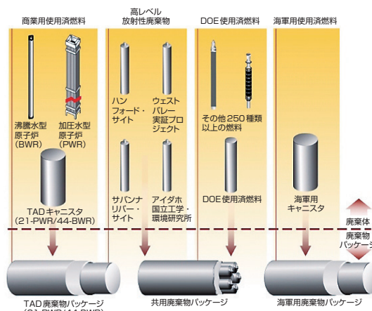
廃棄物パッケージの種類
