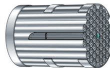
CANDU 炉燃料集合体 180 本をまとめた燃料バスケット
