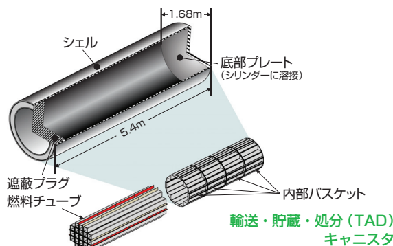
廃棄物パッケージの種類
