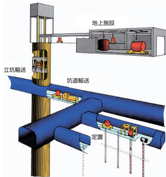
処分坑縦置き方式
