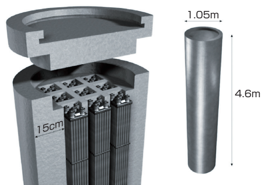
BWRの使用済燃料処分用キャニスタ
