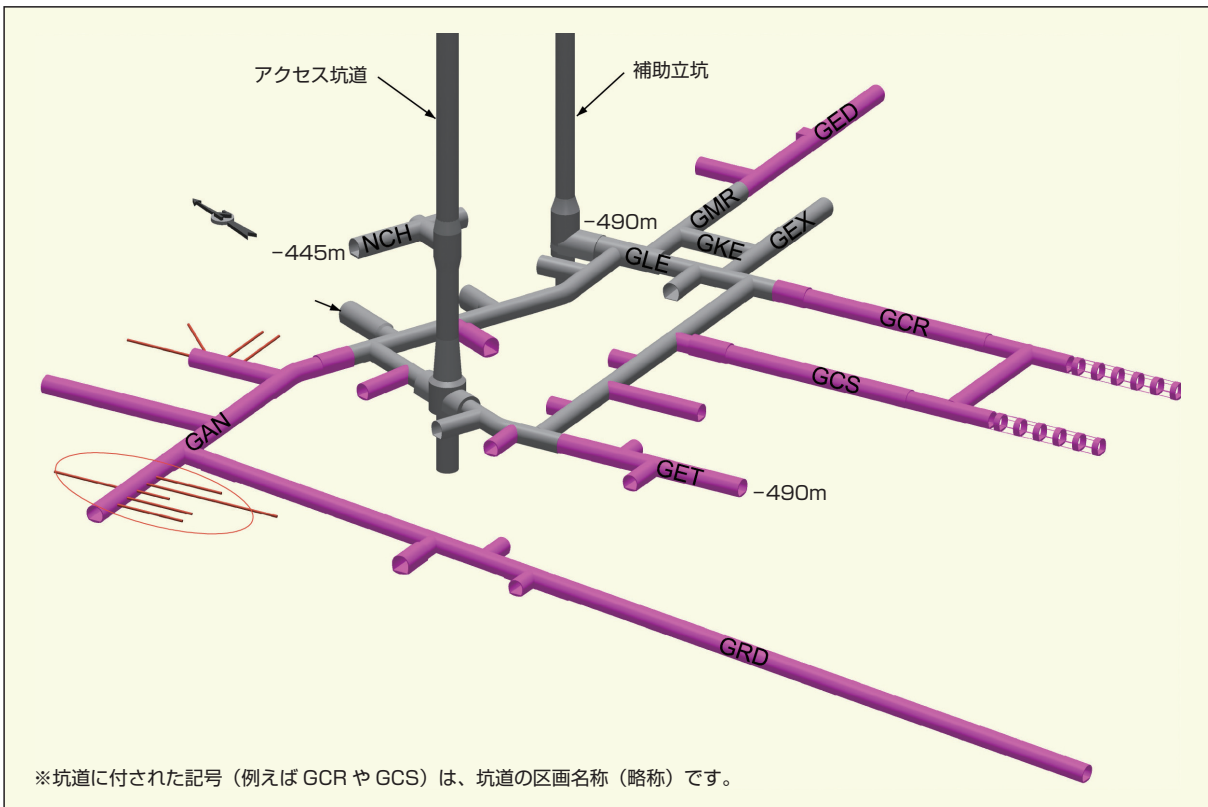
地下研究所の構造 (ANDRA資料より作成)
