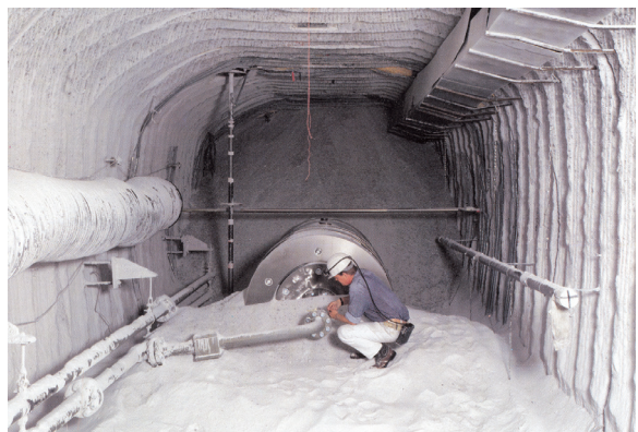
アッセII研究鉱山での実規模キャスクを用いた実験の様相 （写真提供：DBE）
