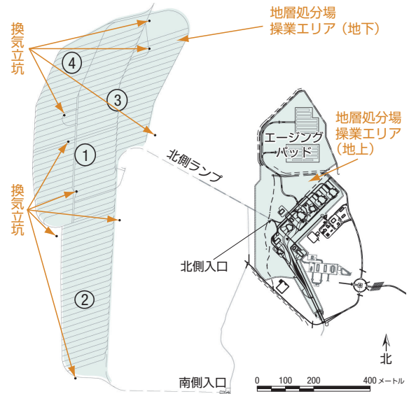
ユッカマウンテン処分場予定地のレイアウト (補足環境影響評価書より引用)
