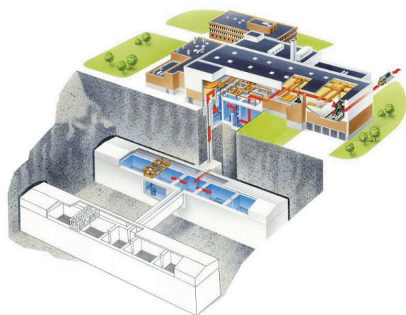
CLAB（使用済燃料の集中中間貯蔵施設）
